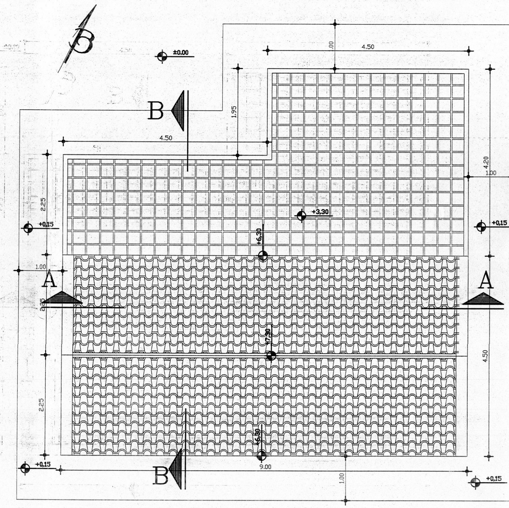
ΚΑΤΟΨΗ ΔΩΜΑΤΟΣ
