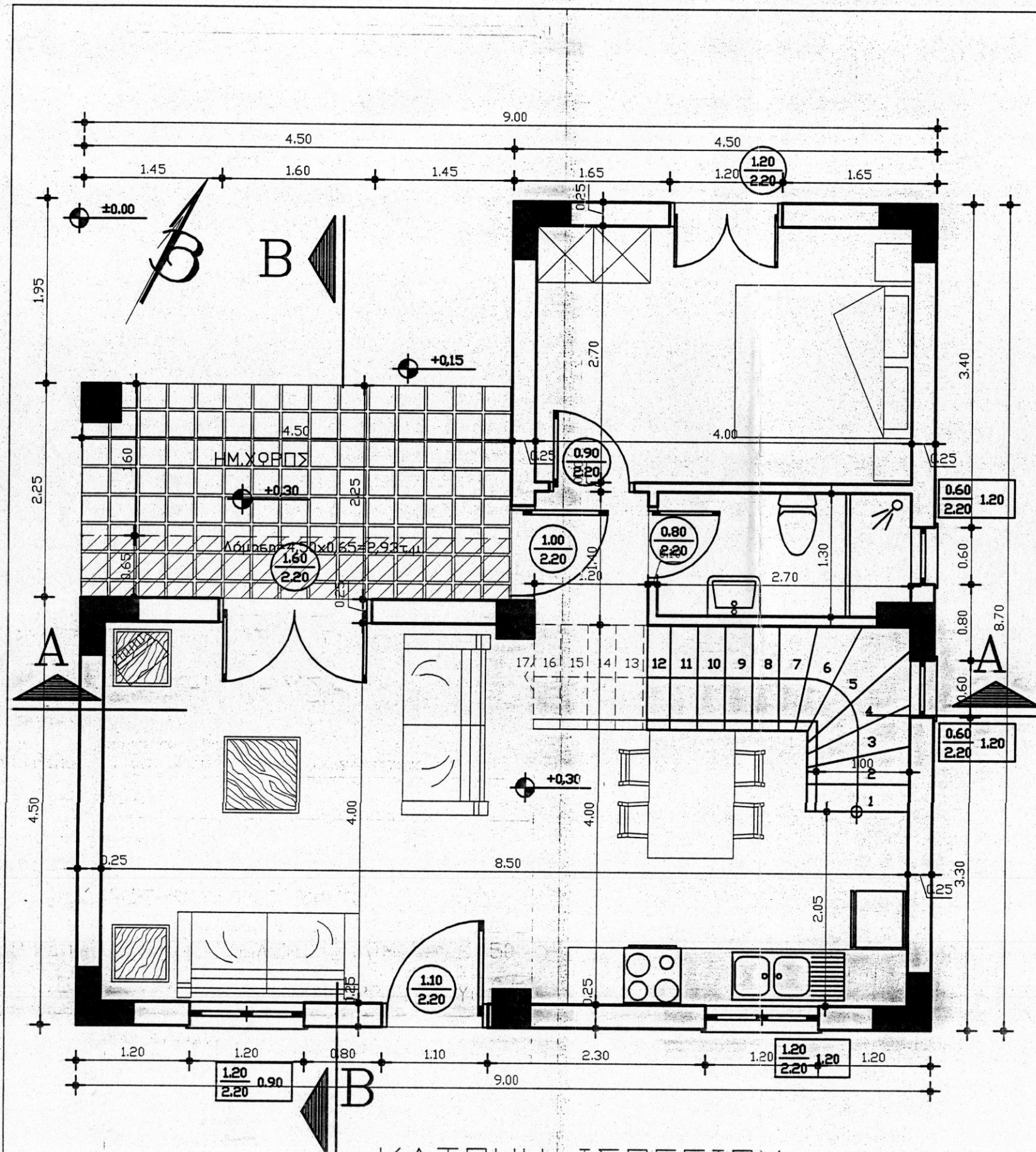
ΚΑΤΟΨΗ ΙΣΟΓΕΙΟΥ
